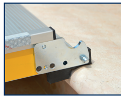
Appoggio al gradino
